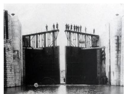
【三池港 (1908 年明治 41 年完成)】完成間近の三池閘門。現在も稼働しています。
